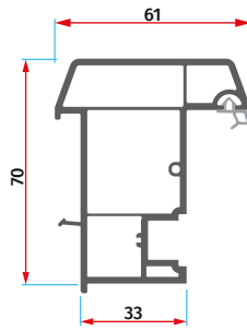
ER 7021 70'lik Hareketli Orta Kayıt Profili 70 Movable Mullion Profile
