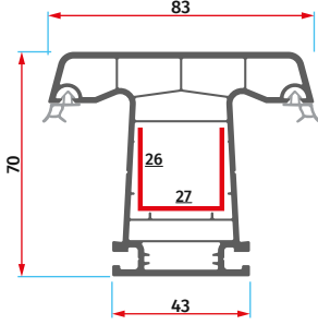
ER 7011 Orta Kayıt Profili Mullion Profile
