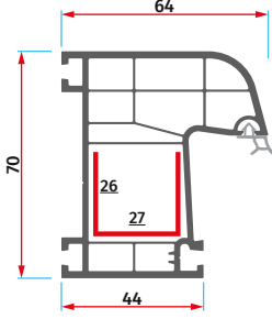
ER 7018 Oval Kasa Profili Ovoid Frame Profile
