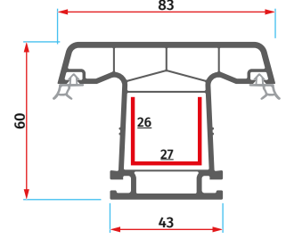
ER 6002 Orta Kayıt Profili Mullion Profile
