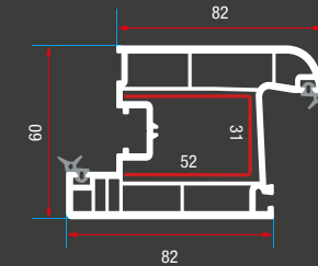
ER 6025 Oval Kapı Kanat Profili ER 6025 Ovoid Door Sash Profile
