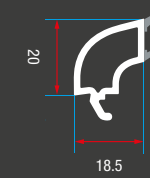
ER 6027 Oval Çift Cam Çıtası ER 6027 Ovoid Double Glazing Bead
