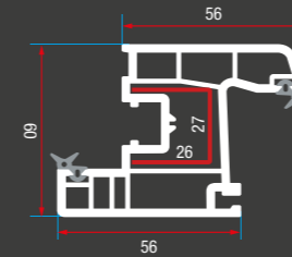
ER 6020 Ekonomik Pencere Kanat Profili ER 6020 Economic Window Sash Profile
