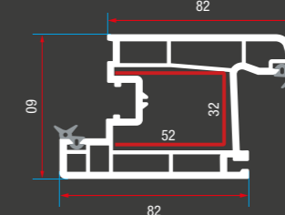
ER 6021 Ekonomik Kapı Kanat Profili ER 6021 Economic Door Sash Profile
